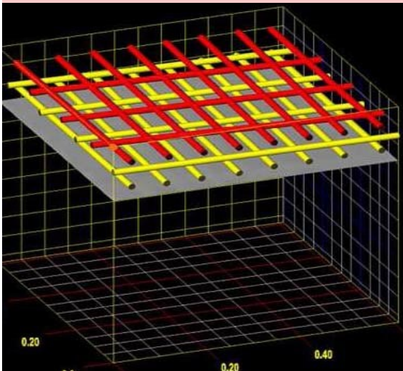
Double Rebar Mat.
